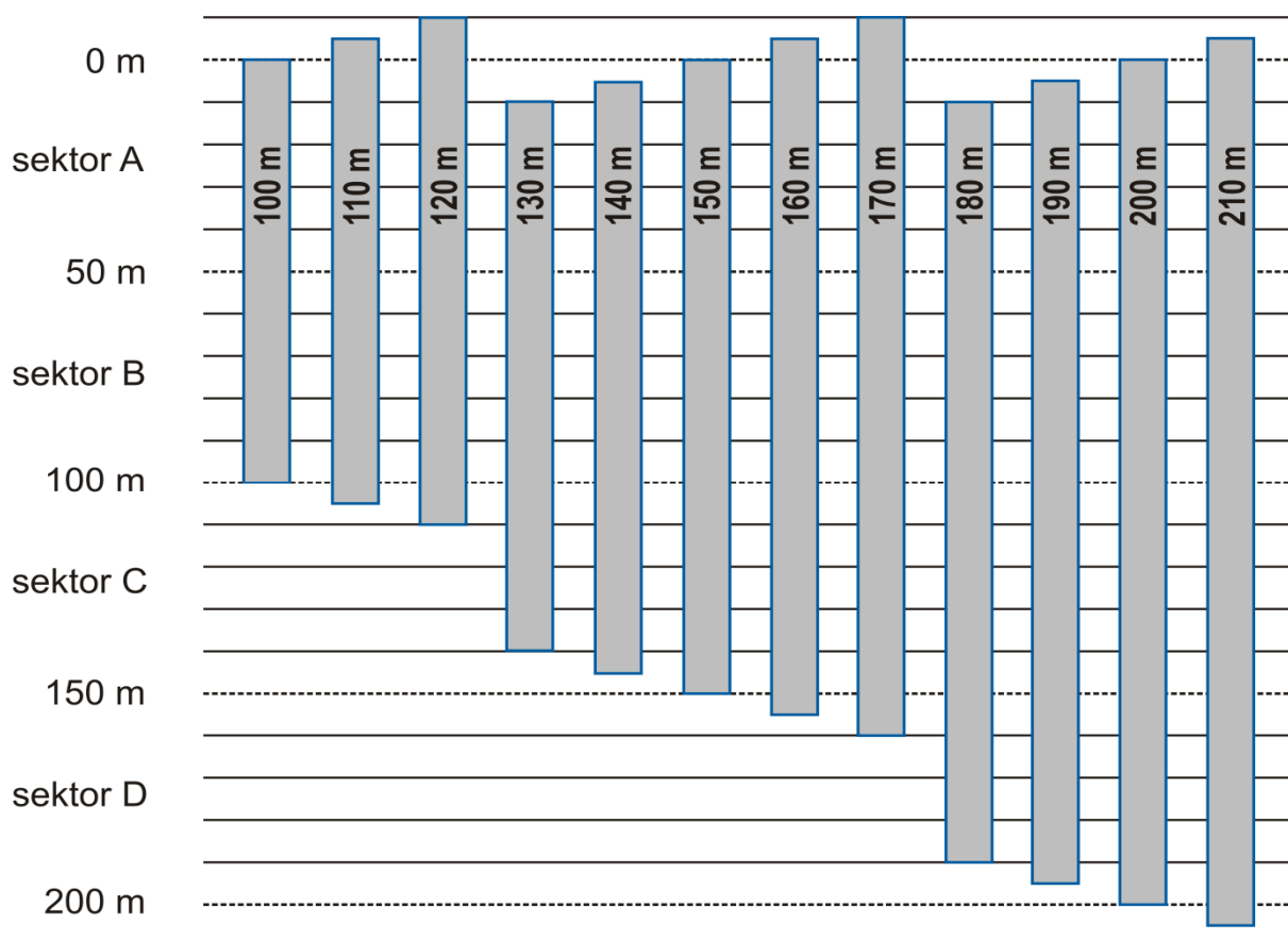
Obr. 1: Princip vyznačení sektorů na nástupištích v závislosti na délce hrany nástupiště (koleje).
