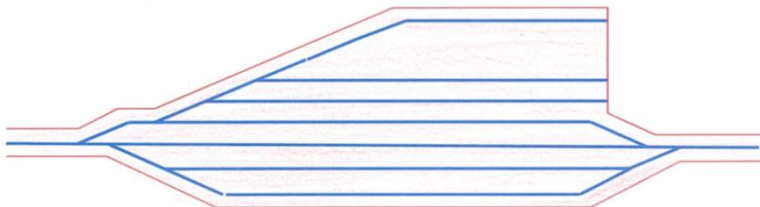
Obr. 4: Zjednodušené grafické vyznačení hranic železniční dopravní cesty v případě dopravy s kolejovým rozvětvením
